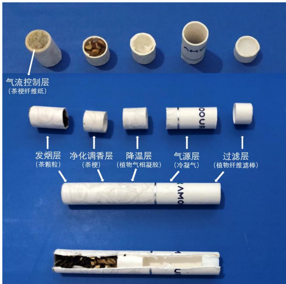
Amour茶叶弹原料构成爆炸图
